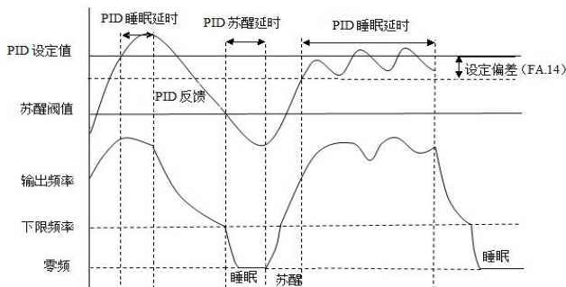
图 FA-6 第二种睡眠模式示意图
