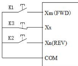
图 F4-4 三线式控制模式 1 示意图
