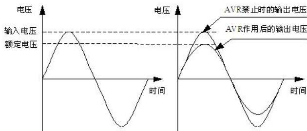
图 FE-2 AVR 功能示意图
