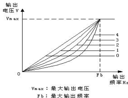
图 F3-1 V/F 曲线示意图
