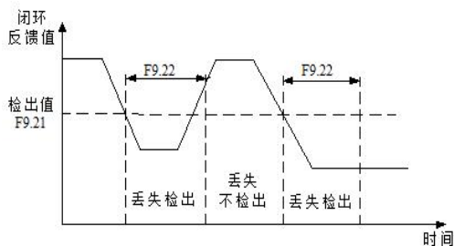
图 F9-4 闭环反馈丢失检出时序图
