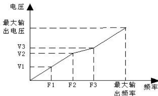
图 F3-4 用户设定 V/F 曲线示意图
