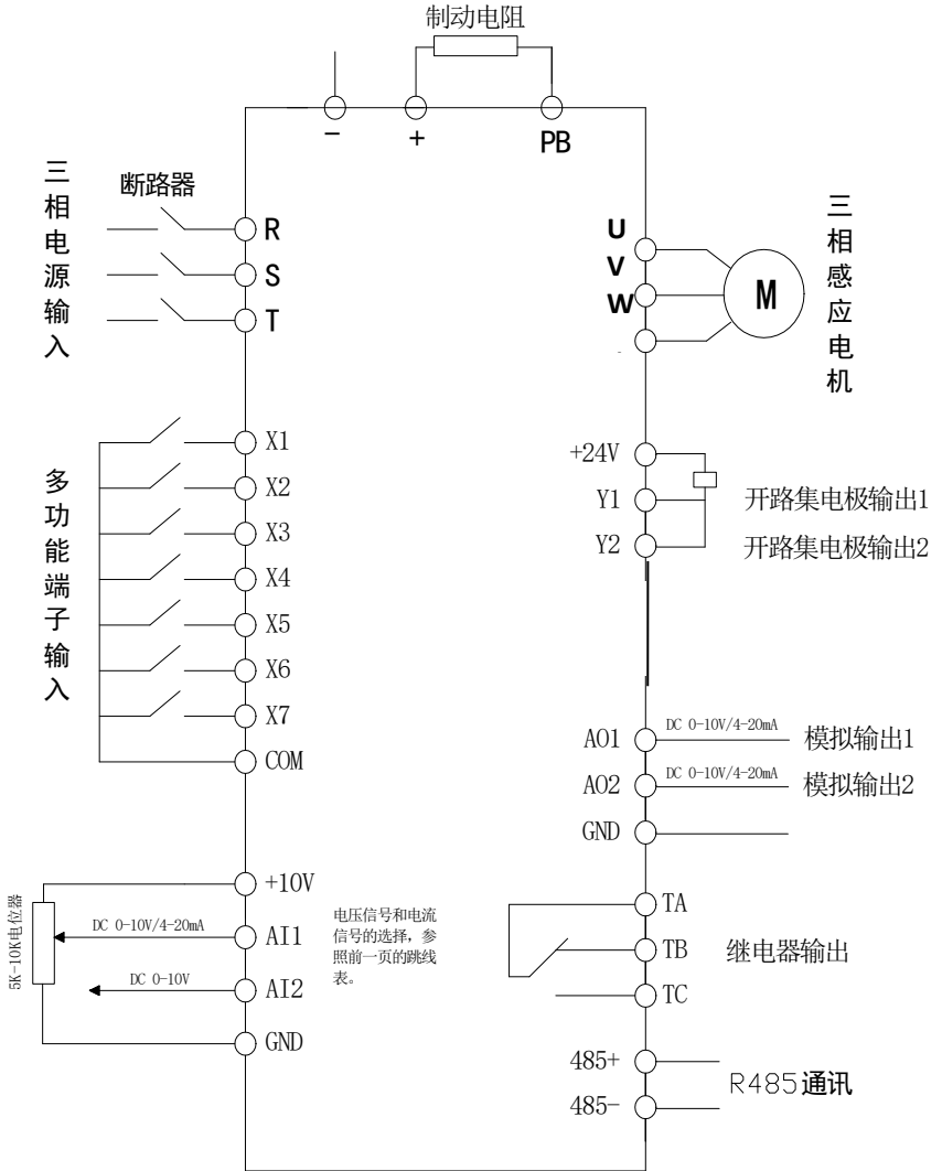
基本运行配线图
