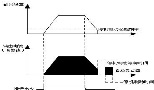
图 F6-4 停机直流制动示意图
