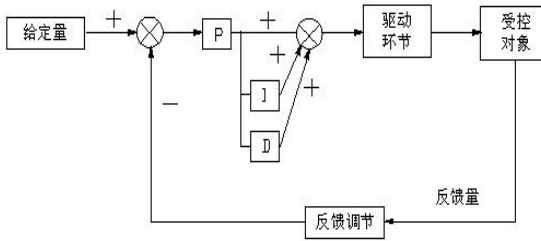
图 FA-2 PID 调节示意图
